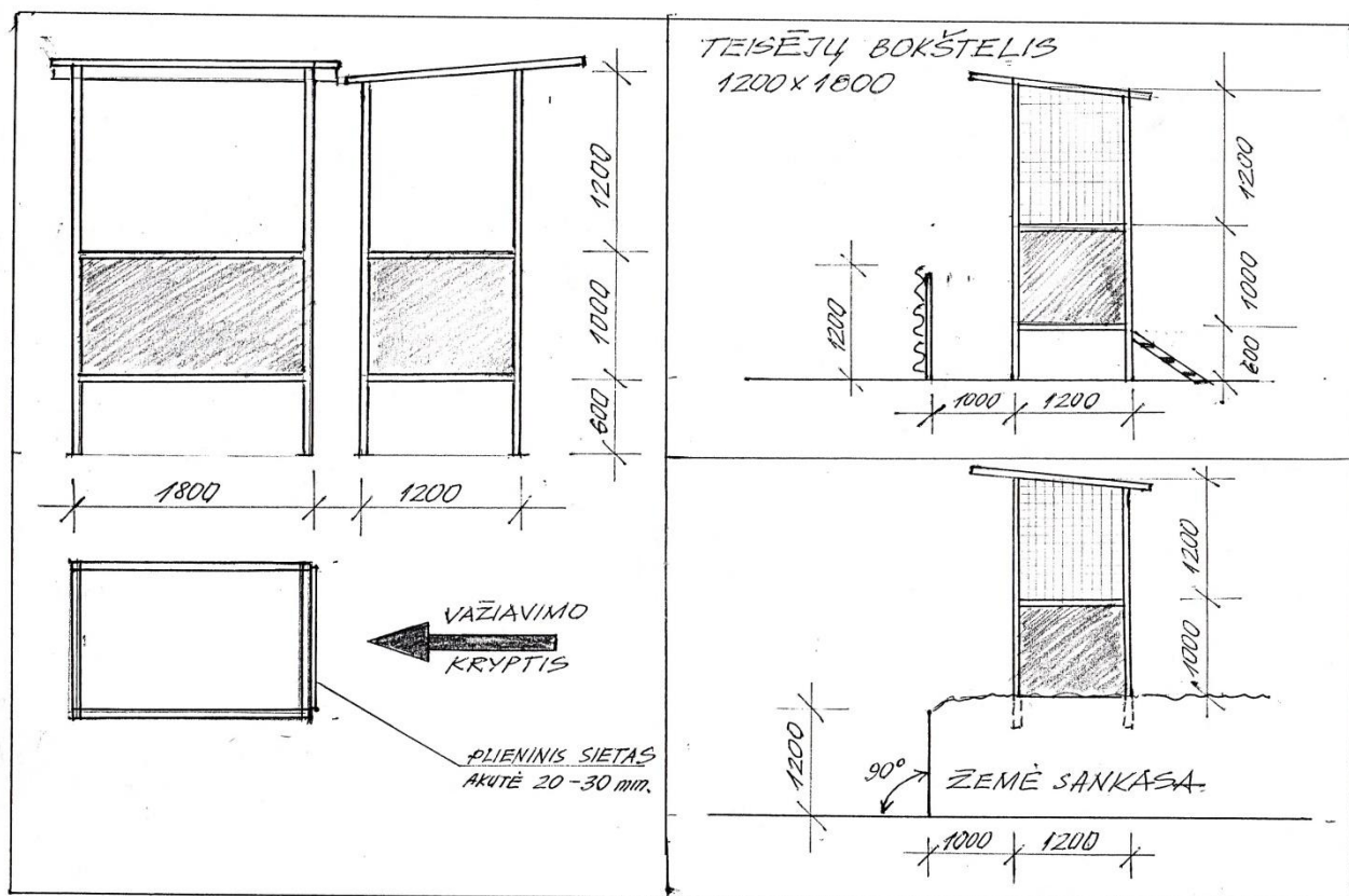
Pav. Nr.2 Teisėjų bokštelio schema
