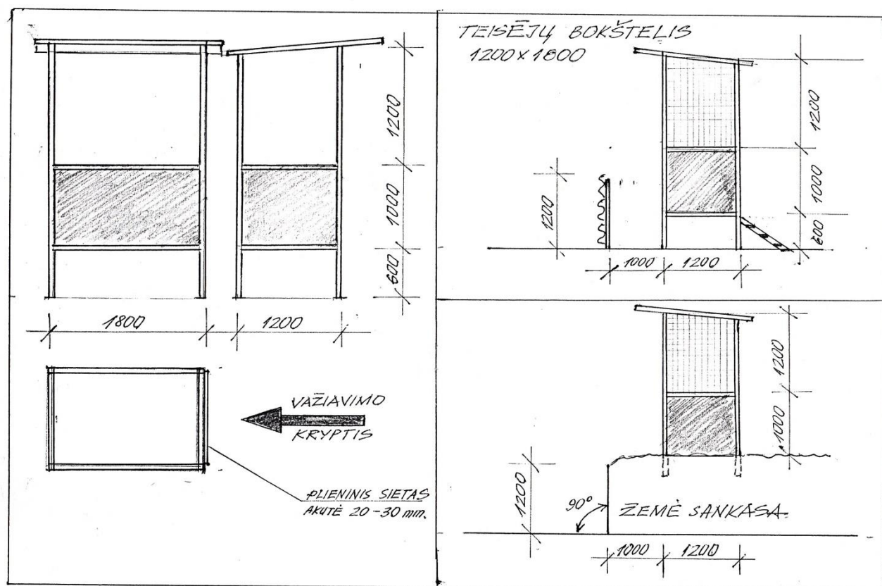
Pav. Nr.2 Teisėjų bukštelio schema
